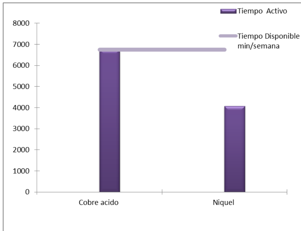
Gráfico 1 Capacidad de la línea Compartida a 2013
