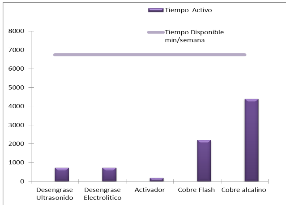
Grafico 26 Capacidad proyectada de la línea Lead Free 2012
