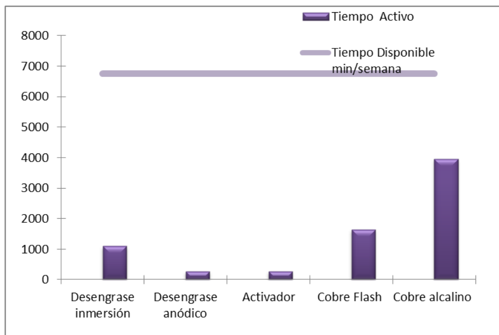
Grafico 25 Capacidad proyectada de la línea Zamac 2012
