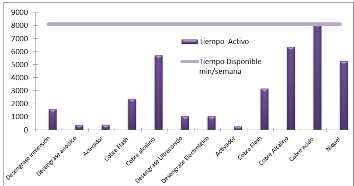
Gráfico 4 Tiempos activos de las líneas de Zamac, Lead Free y MP a 2015
