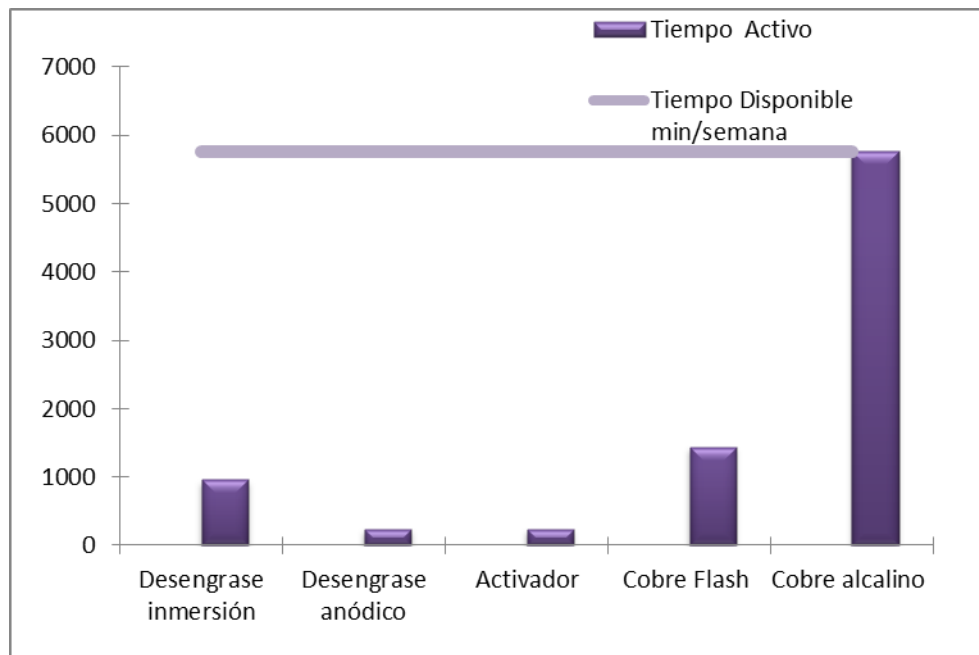
Grafico 23 Capacidad Actual De La Línea Zamac
