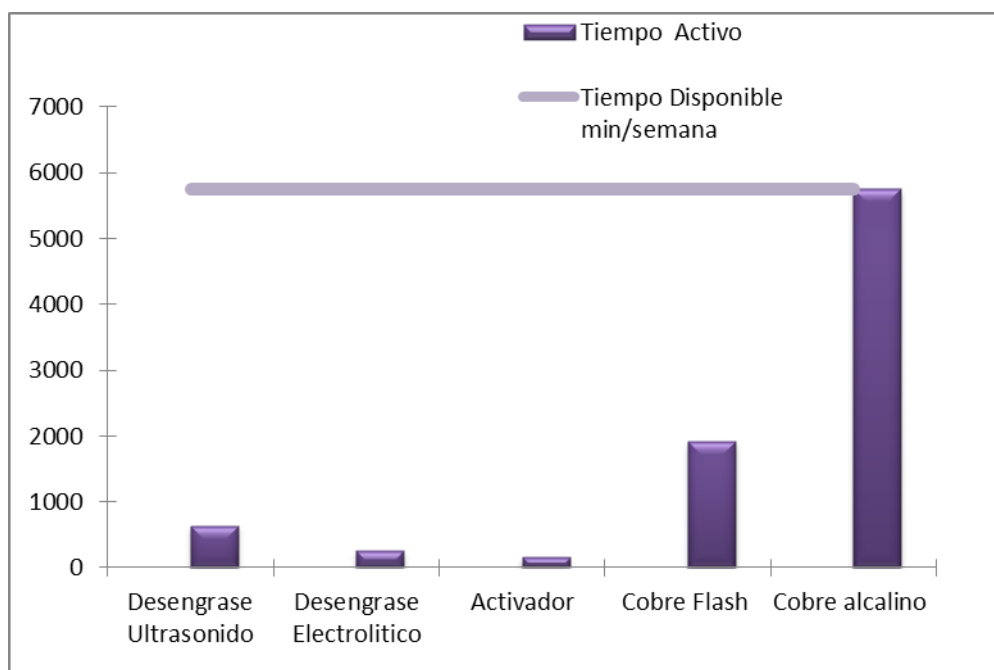
Grafico 18 Tiempos activos de la línea de Lead Free y MP
