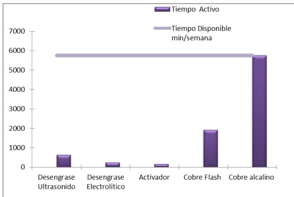
Grafico 24 Capacidad actual de la línea de Lead Free y MP
