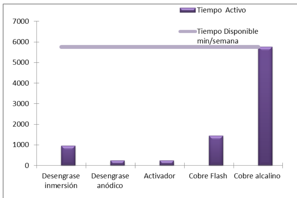
Grafico 17 Tiempos activos de la línea de Zamac
