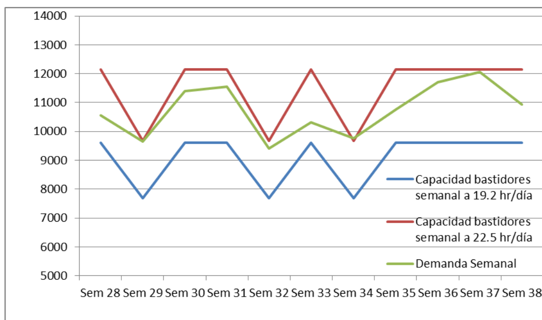
Grafico 22 Capacidad a 19.2 hr y 22.5 hr diarias y demanda actual año 2012 semanalmente. Con ampliación del tanque de cobre alcalino
