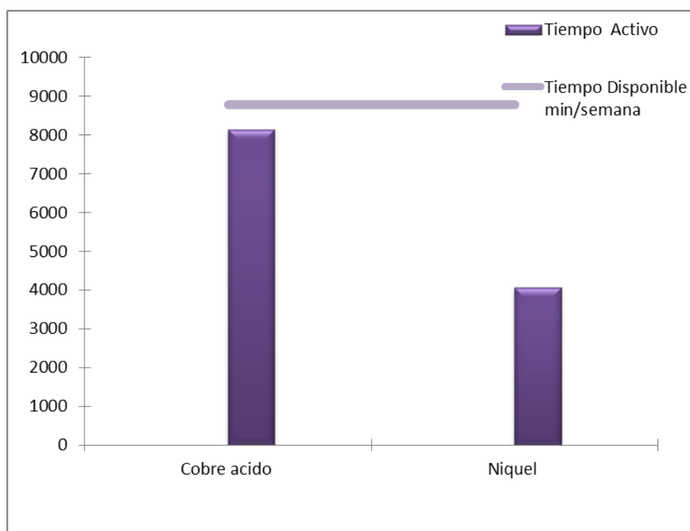
Gráfico 2 Tiempo activo proyectado de la línea compartida de cobre ácido y níquel a 2013
