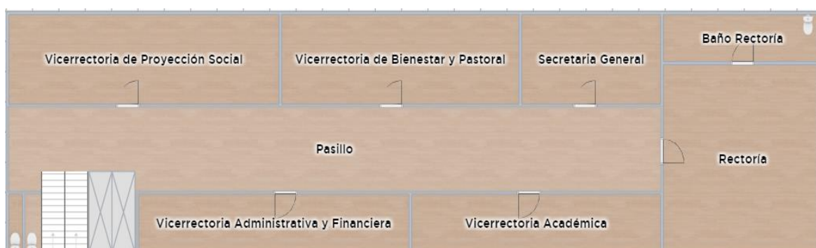
Figura 23. Distribución de espacios piso 5 Fundación Universitaria San Gabriel.
